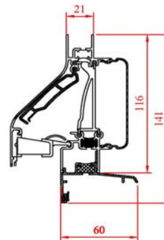
DUCOKLEP 25/Aanslag BI
