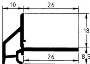
condensprofiel 7mm
