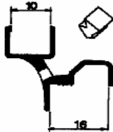
condensprofiel 10mm
