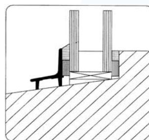
ventilerend onderprofiel laag (= stooltjes profiel)
