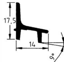
ventilerend onderprofiel laag (= stooltjes profiel)
