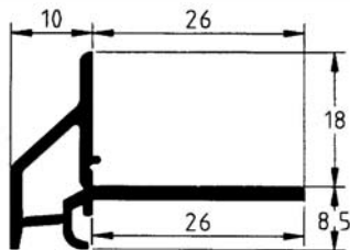
condensprofiel 7mm
