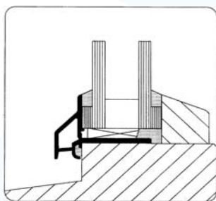
binnenbeglazingsprofiel (= L profiel)
