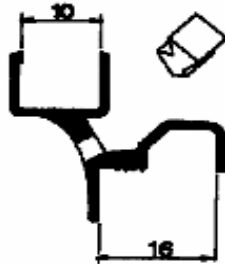
condensprofiel 10mm
