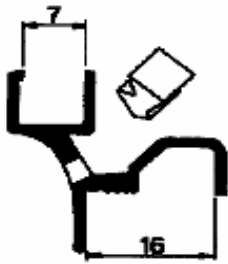
condensprofiel 7mm
